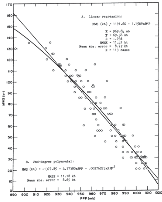
Figure 7 V_{max} vs p_c : WNP : data.
